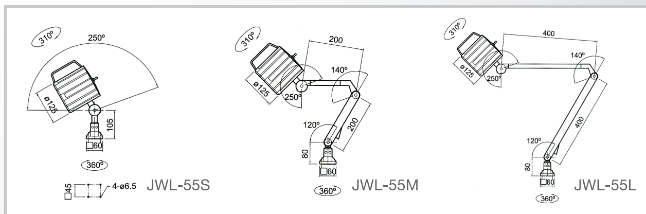
JWL-55L DŁUGIE RAMIĘ
